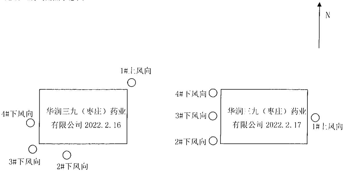
无组织废气测点示意图
